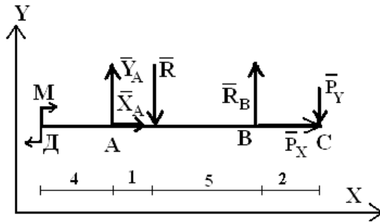
Рис. 7. Расчетная схема
