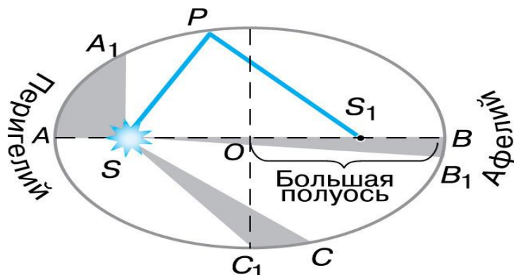
Рис. 2 Свойства эллипса
