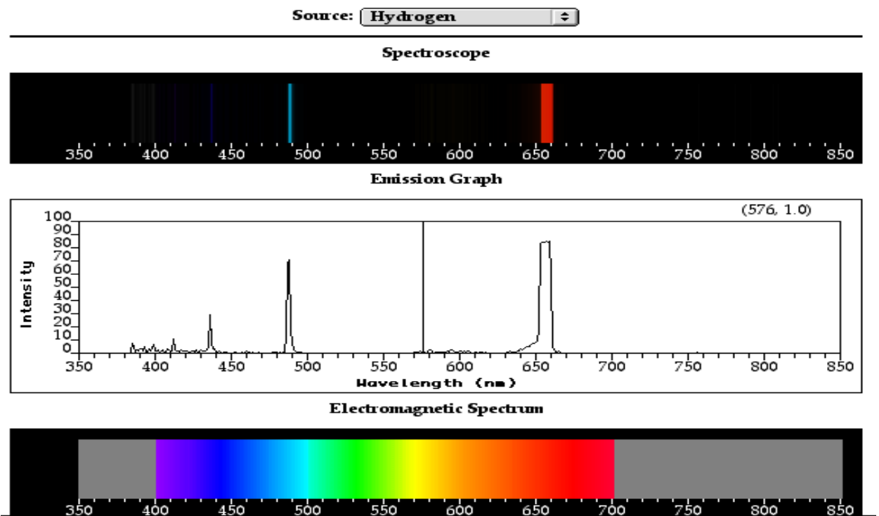
Рис. 1 Спектр водорода
